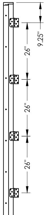
HINGE JAMB
