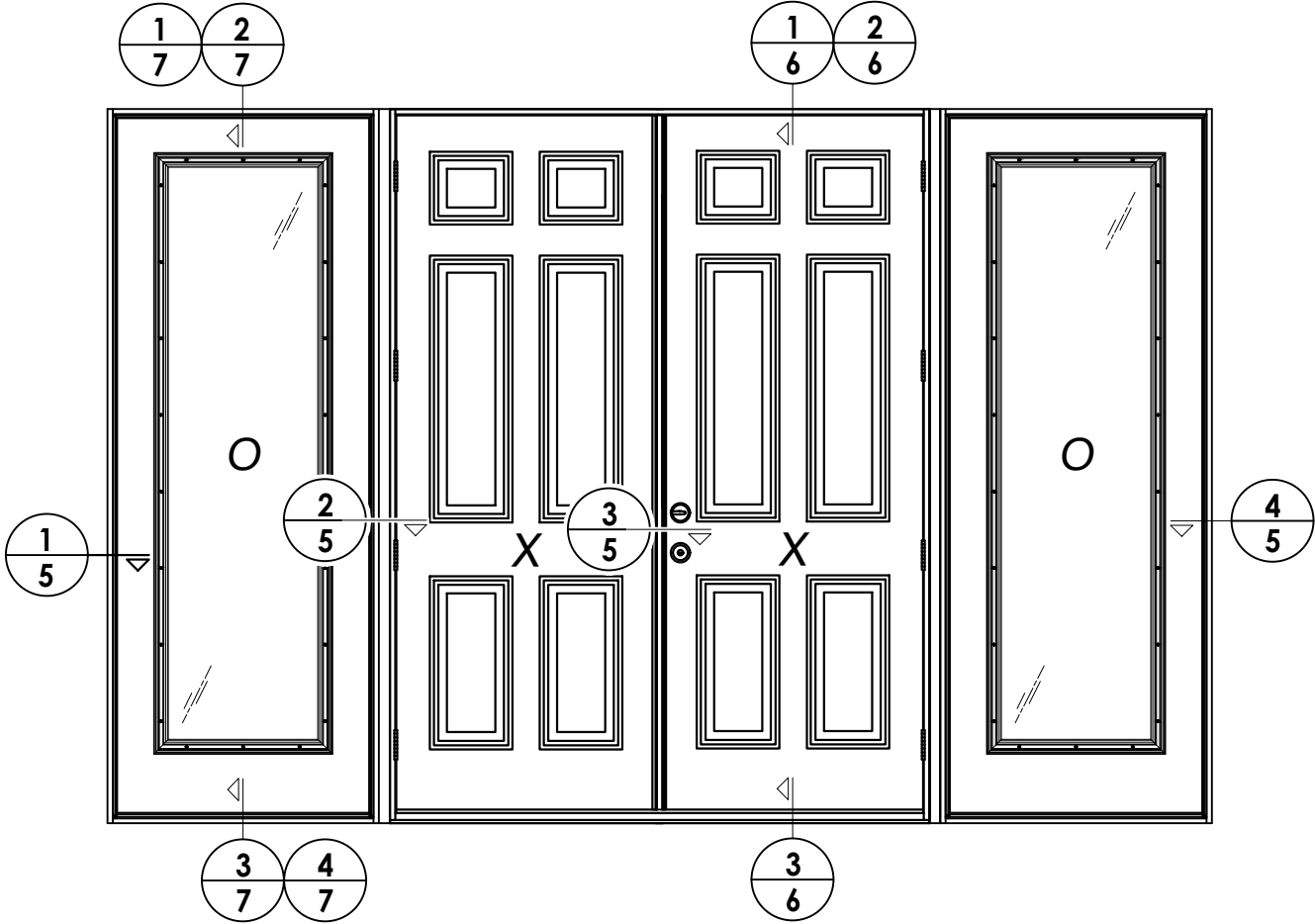
ELEVATION (OXXO)
